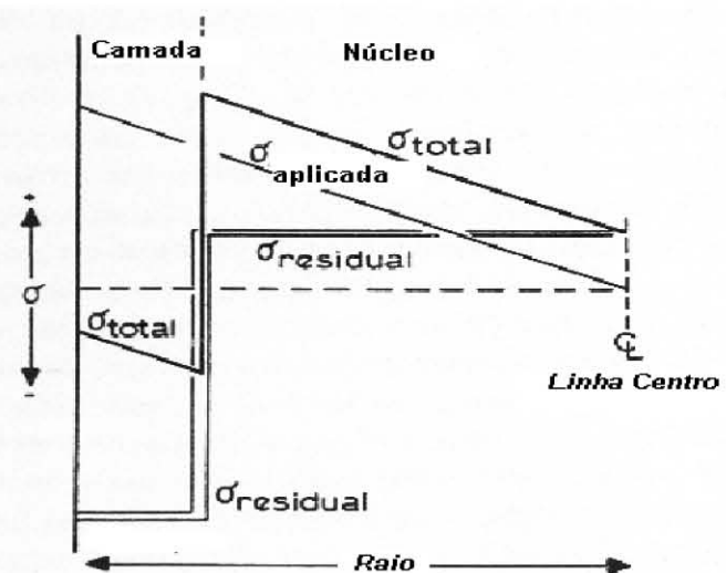
Figura I. Distribuição de tensões numa mola (4)
