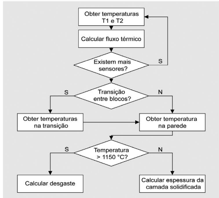
Diagrama I. Fluxo de cálculo do desgaste do cadinho
