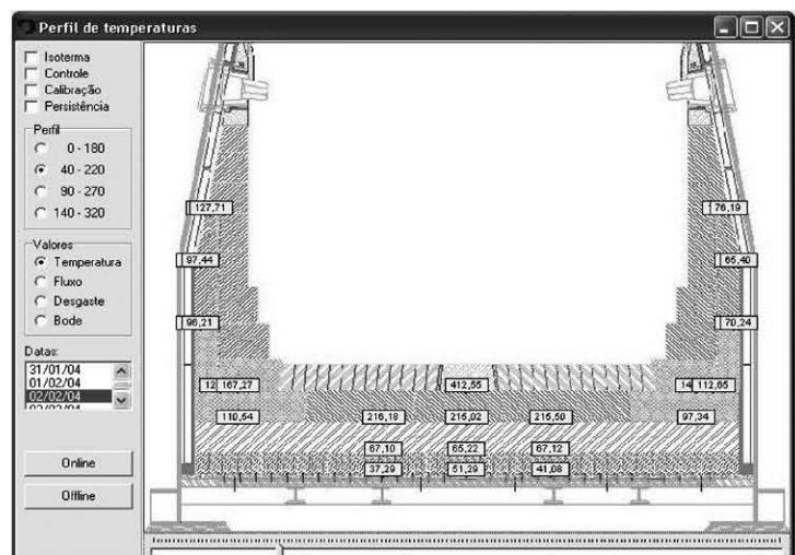
Figura 3. Tela de visualização do perfil do cadinho
