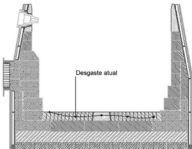
Figura 4. Perfil atual de desgaste.
