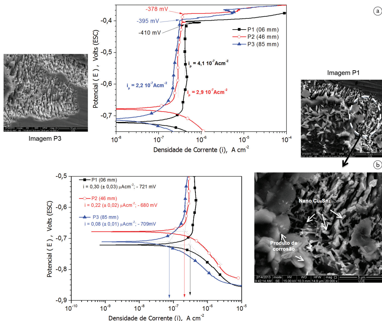
Figura 7. (a) Curvas experimentais de polarização evidenciando as regiões anódicas e imagens por MEV das microestruturas nas posições P1 e P3 e (b) curvas experimentais evidenciando as linhas de extrapolação Tafel para obtenção das densidades de corrente de corrosão.
